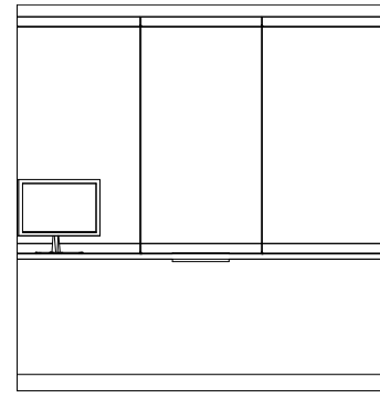
3 A983 OPTION - B 1/4" = 1'-0"
